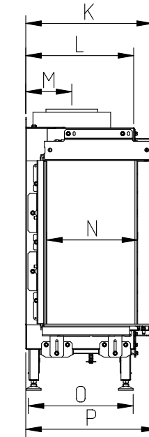
Right Elevation
