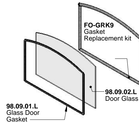
99.09.02.L Door Glass & Gasket
