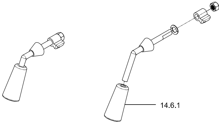
99.09.04.N DOOR HANDLE ASSEMBLY
