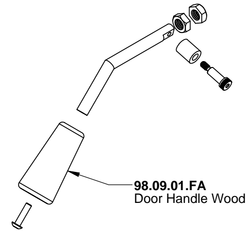
ER-99.09.01.FA Door Handle Assembly
